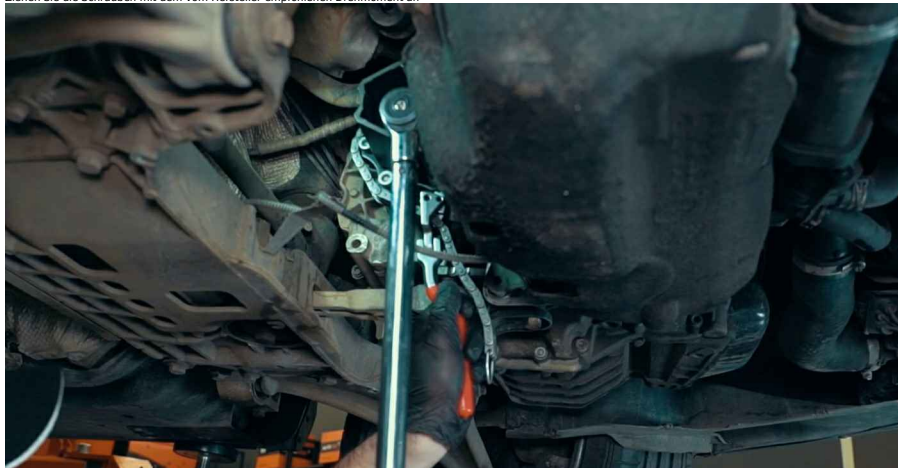
13 Falls die Antriebswelle in das Differential eingesetzt wurde, muss zunächst das Getriebeöl abgelassen werden
