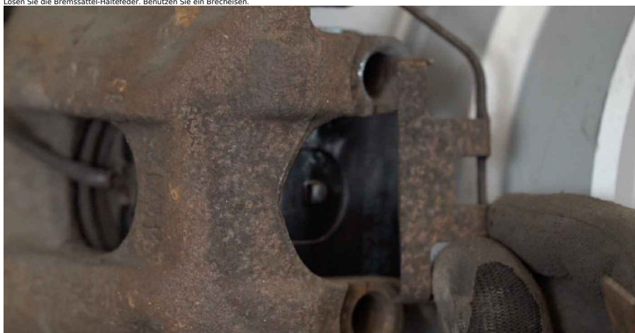
14 Entfernen Sie den Bremssattel.
